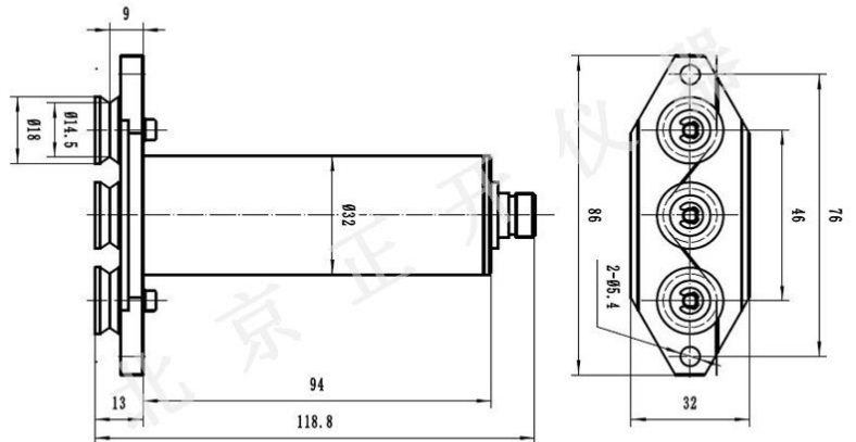
外形尺寸图
