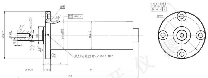
外形尺寸图
