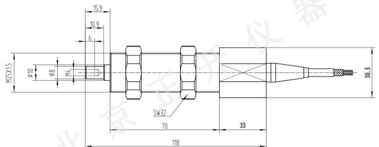
MCL-T31型电缆线为尾部出线，轴端尺寸默认 \phi 8 \times 10.9 ，可以按需订制
