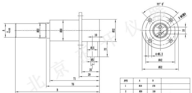
外形尺寸图
