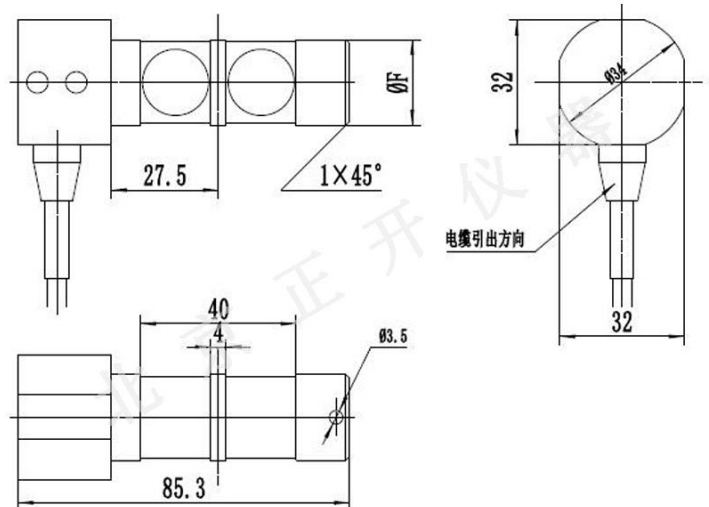
外形尺寸图
